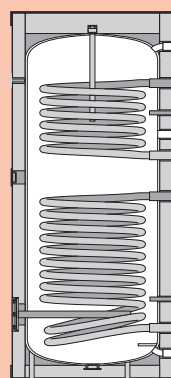
V2 – dva výměníky
