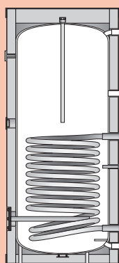
V1 – jeden výměník
