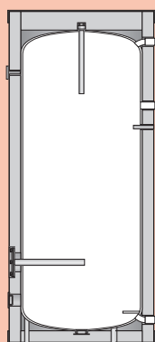
V0 – bez výměníku
