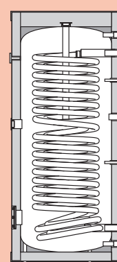
V3 – tři výměníky
