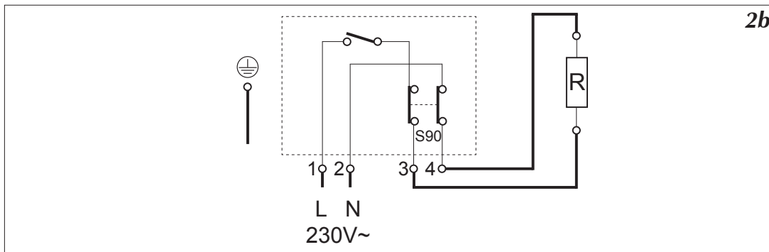
Obr.2b Schéma elektrického zapojení pro ohřívače FPD 10
