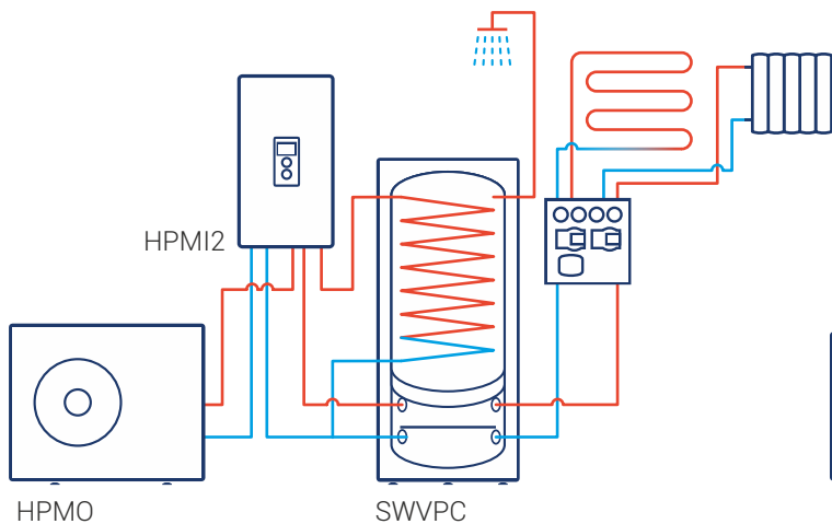
Instalace systému – sestava HPM.V - ilustrační schéma
