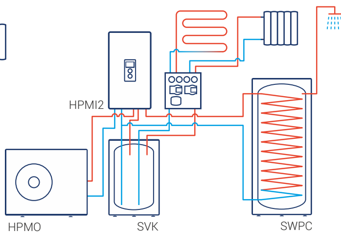
Instalace systému – sestava HPM.P - ilustrační schéma
