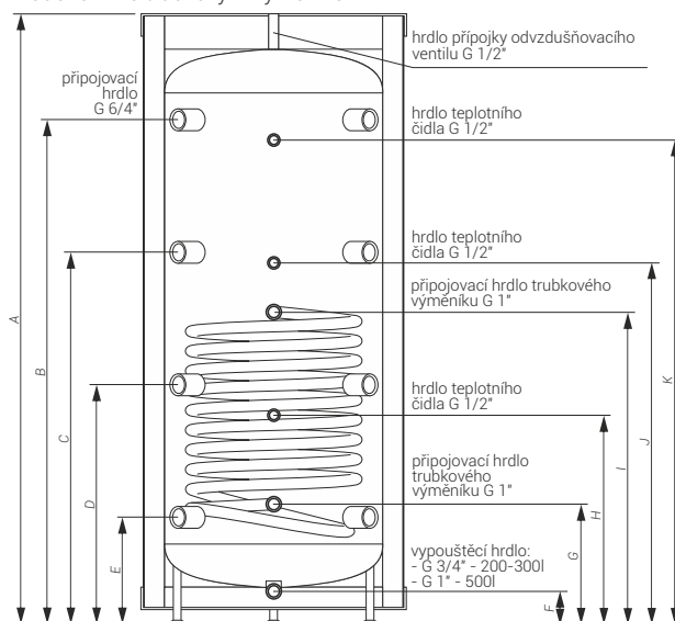
model SVW s trubkovým výměníkem
