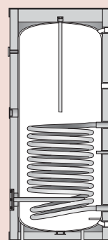
V1 – jeden výměník
