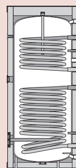
V2 – dva výměníky
